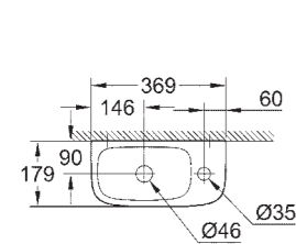
39 327 000 39 327 00Н* Компактная мини-раковина 37 см
