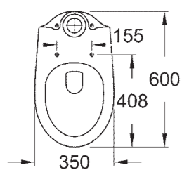
39 428 000 Унитаз приставной, горизонтальный выпуск
