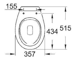
39 431 000 Унитаз напольный, вертикальный выпуск
