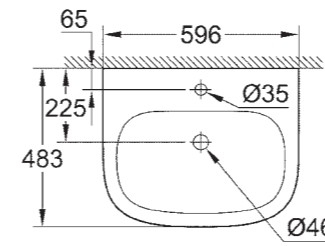
39 337 000 39 337 00Н* Встраиваемая раковина 60 см
