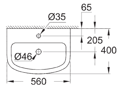
39 422 000 Раковина встраиваемая сверху 55 см
