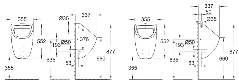
39 438 000 Писсуар, скрытый монтаж
