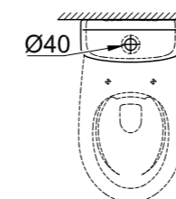
39 429 000 Унитаз приставной, вертикальный выпуск
