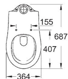
39 429 000 Унитаз приставной, вертикальный выпуск
