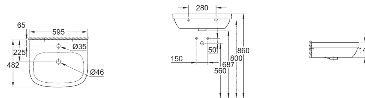
39 335 000 39 335 00H* Раковина подвесная 60 см
