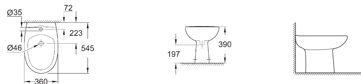
39 432 000 Биде напольного монтажа
